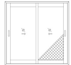
2.5T 2S + Mesh
